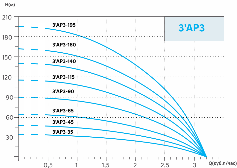
рисунок 1. График напорных характеристик
